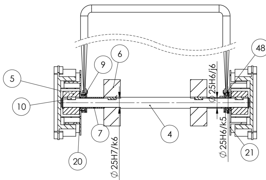
B-B M 1:5
