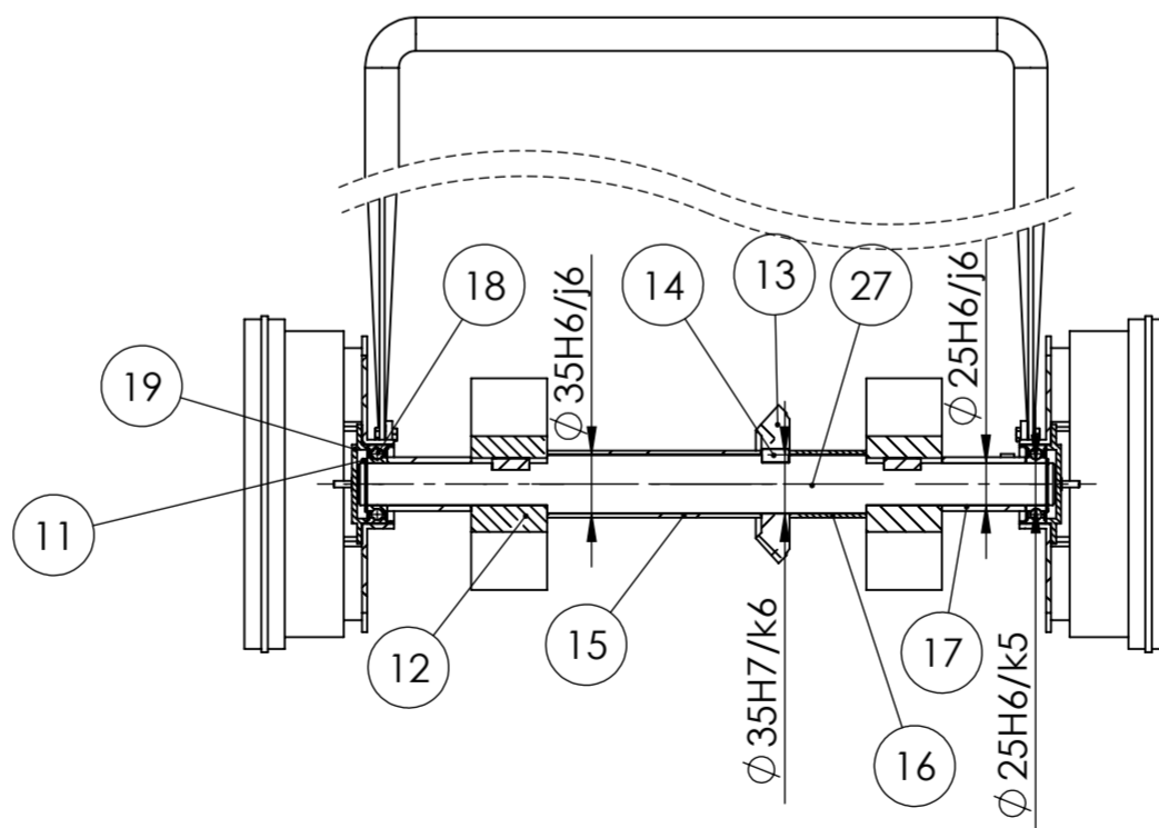
B-B M 1:5
