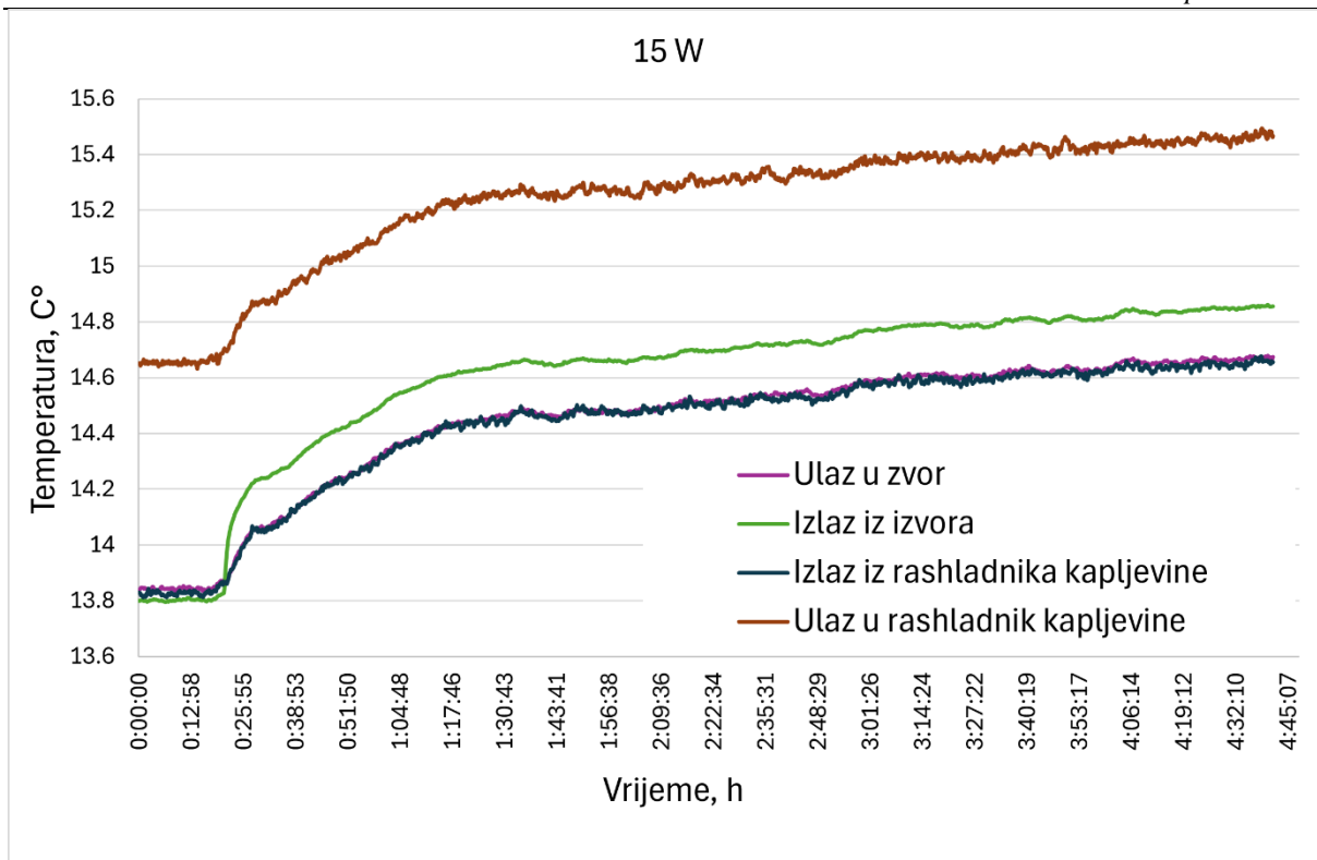
Slika 27 Promjena temperature rashladne smjese u vremenu za snagu CT uređaja od 15 W
