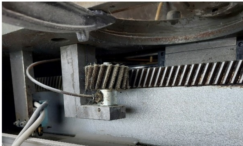
Slika 24. Spužvasti zupčanik za podmazivanje pogonskog zupčanika i zubne letve
