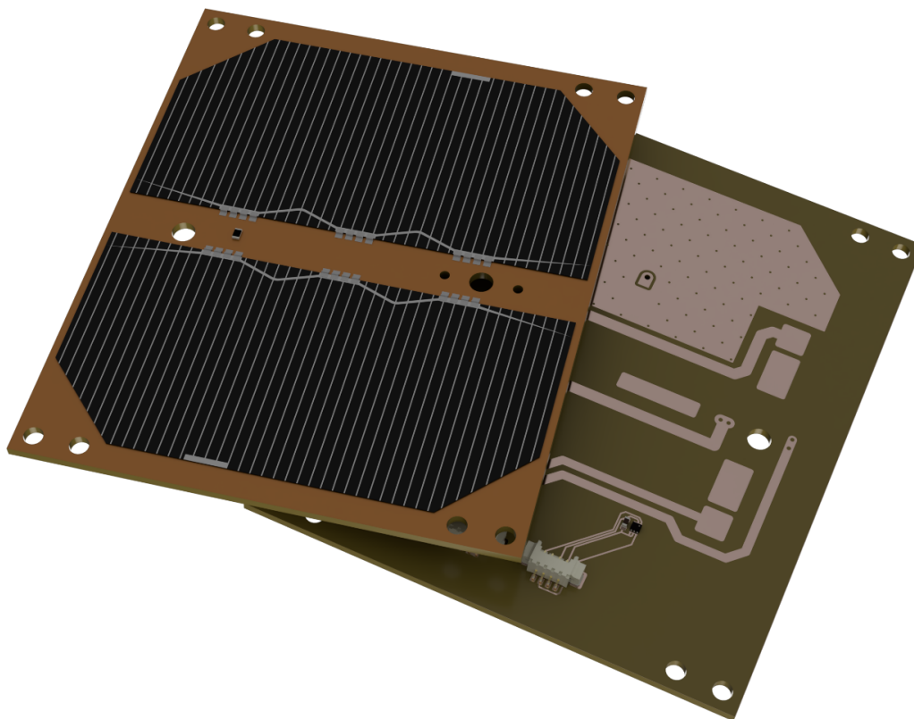
Slika 15. Solarni paneli
