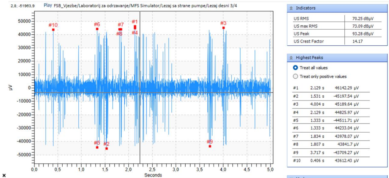
Slika 35. Vremenska domena signala ležaja s oštećenom kuglicom
