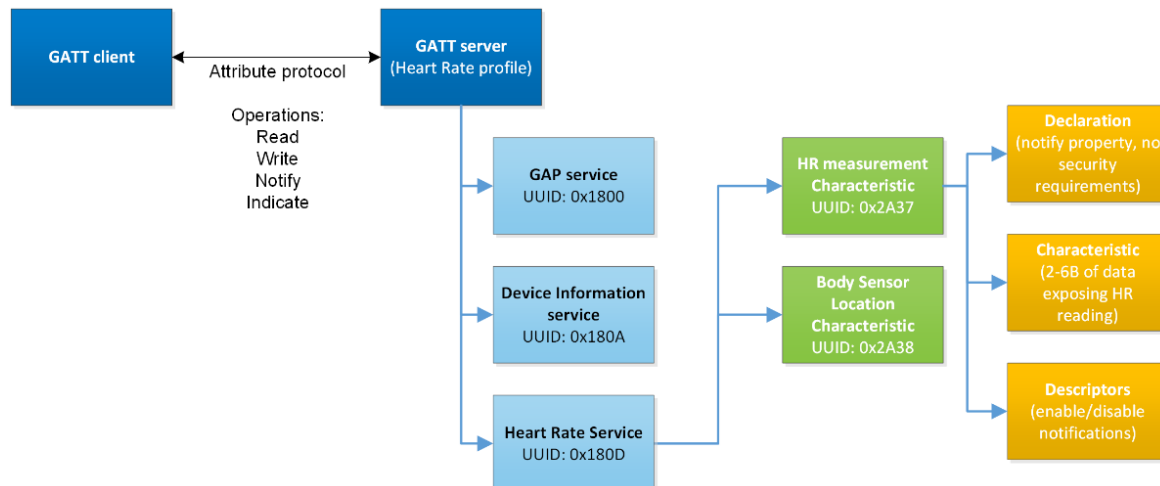
Slika 24. Struktura GATT [38]
