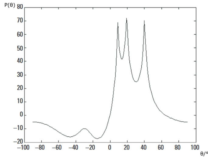
Slika 40. Estimacija DOA s MUSIC algoritmom, smjerovi radio signala su 10°, 20° i 40° [46]
