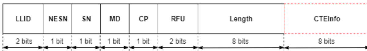
Slika 29. Zaglavlje PDU fizičkog kanala podataka [41]
