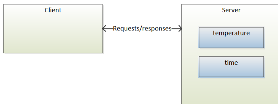
Slika 22. Uloge uređaja [38]
