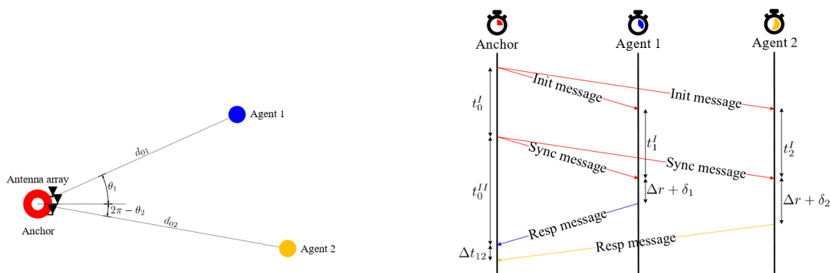
Slika 14. AoA + ToF [28]
