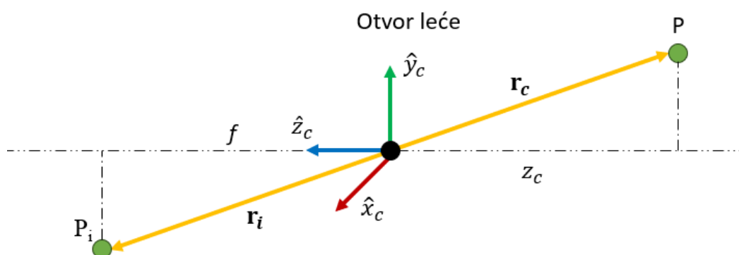
Slika 2.3. Određivanje jednačbi perspektivne projekcije
