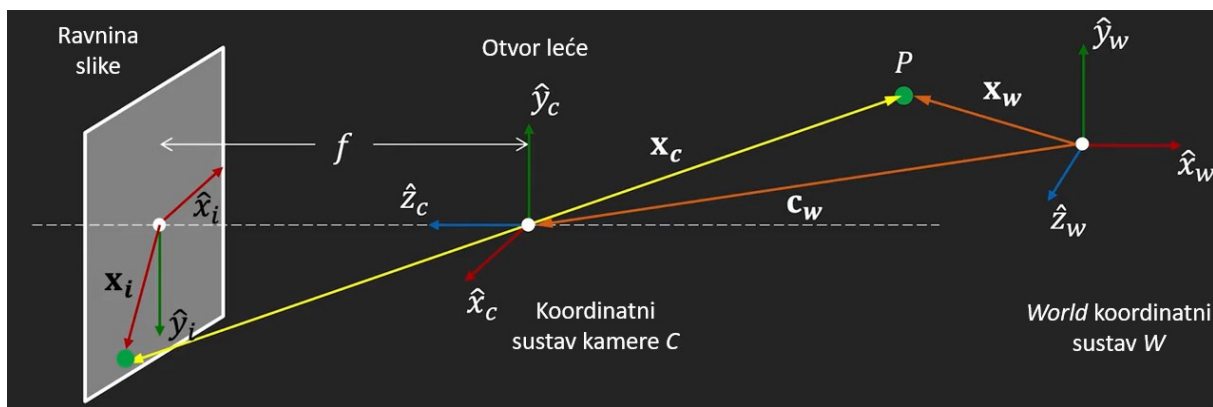
Slika 2.2. Pinhole model kamere [9]
