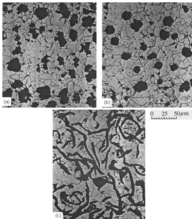
Slika 14. Tipična struktura triju željeznih ljevova (a) Crni temper (kovkasti) ljev (3.1 % C, 2.39 % Si, 0.37 % Mn), HB 150. (b) Nodularni (žilavi) ljev (3.1 % C, 2.41 % Si, 0.43 % Mn), HB 150. (c) Sivi željezni ljev (3.2 % C, 2.43 % Si, 0.32 % Mn), HB 105. [10]
