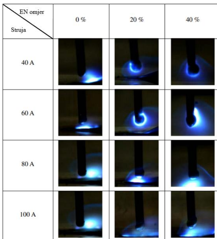
Slika 18. Formiranja kapljica s različitim EN omjerom i različitim strujama zavarivanja [14]
