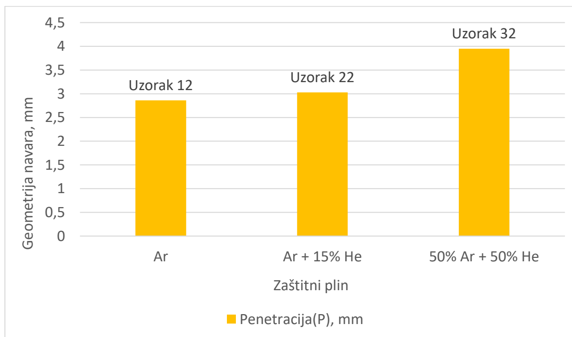
Slika 67. Graf ovisnosti penetracije navara o udjelu He u zaštitnom plinu (EN = 0%)
