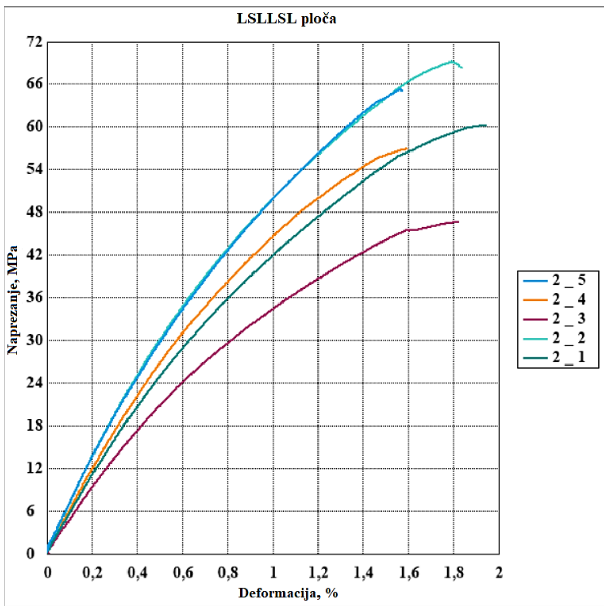
Slika 27. Dijagrami rastezno naprezanje-istezanje za LSL/SL ploču
