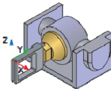
Slika 6.4. Zakrenuti koordinatni sustav – obrada druge bočne stranice [12]
