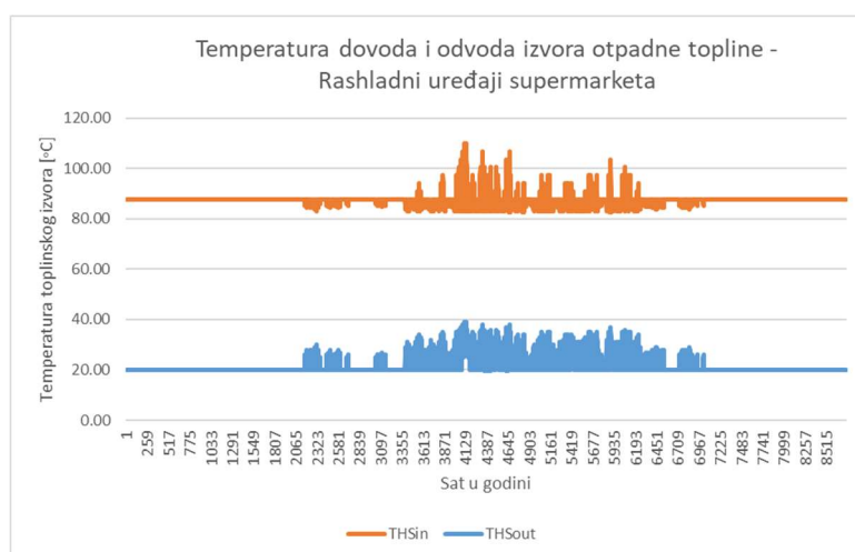
Slika 13: Temperature odvoda i izvoda Rashladnih uređaja samoposluga
