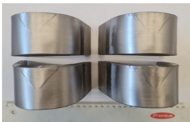
Slika 43. Izgled lica i korijena zavara nakon savijanja
