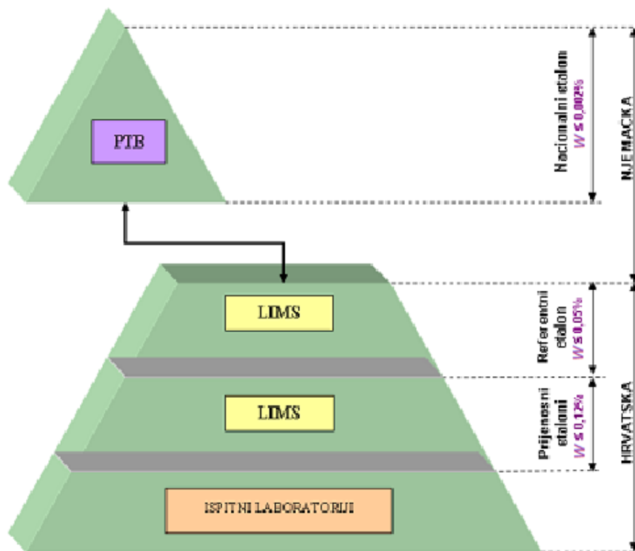
Slika 3. Piramida sljedivosti mjerila sile [14]
