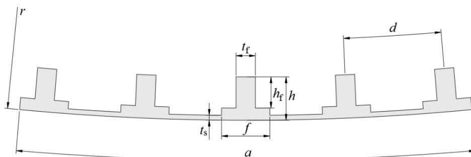
Slika 21. Geometrijski parametri panela
