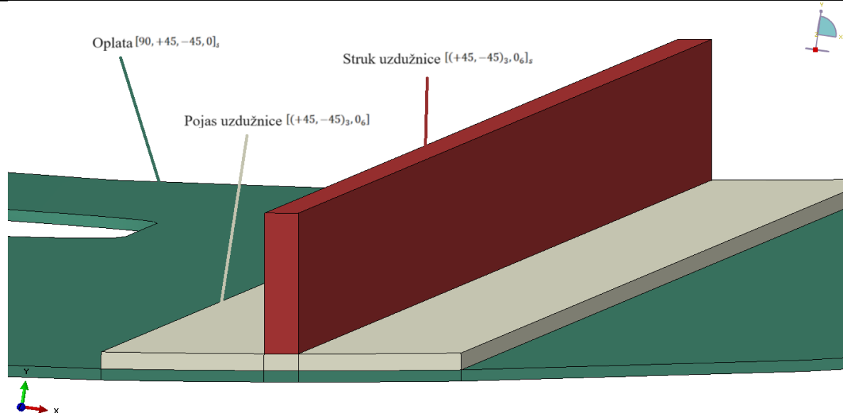
Slika 23. Raspored slojeva po dijelovima konstrukcije
