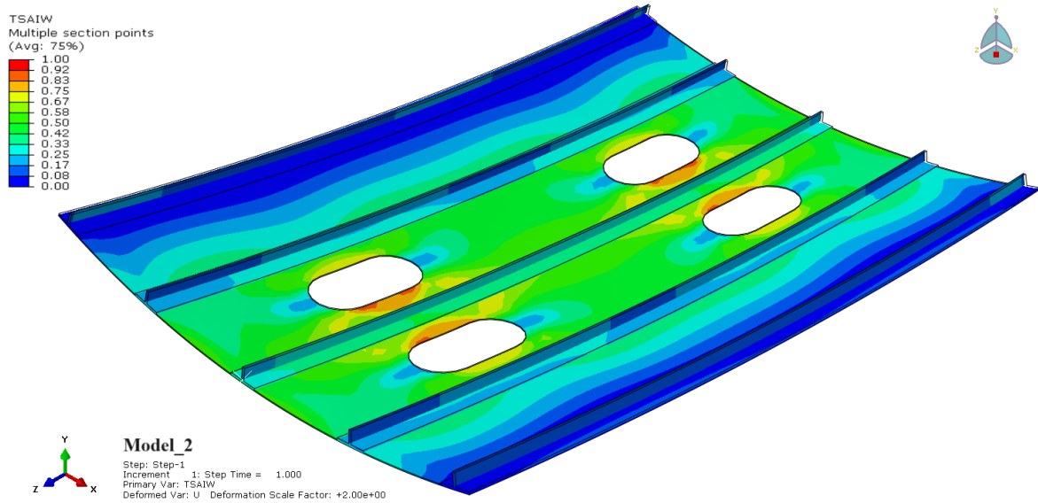
Slika 29. Tsai-Wu kriterij
