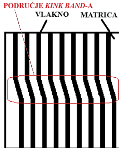
Slika 7. Izvijanje vlakna
