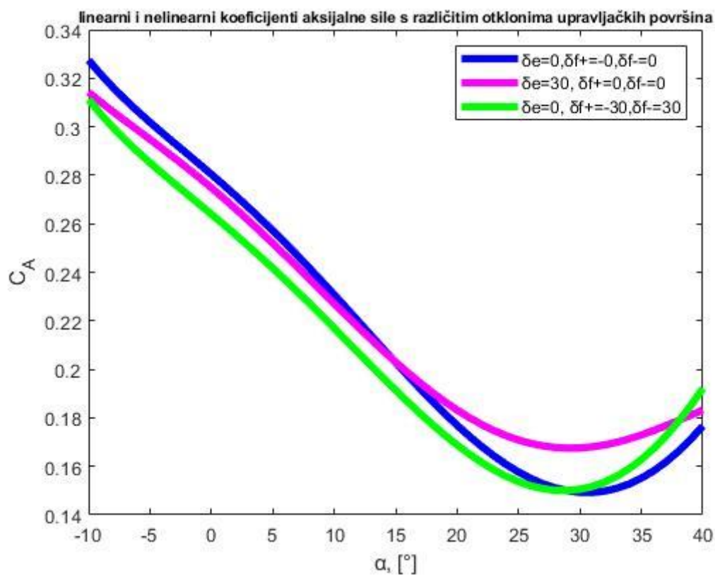
Slika 10. Grafički prikaz ovisnosti koeficijenta aksijalne sile o napadnom kutu
