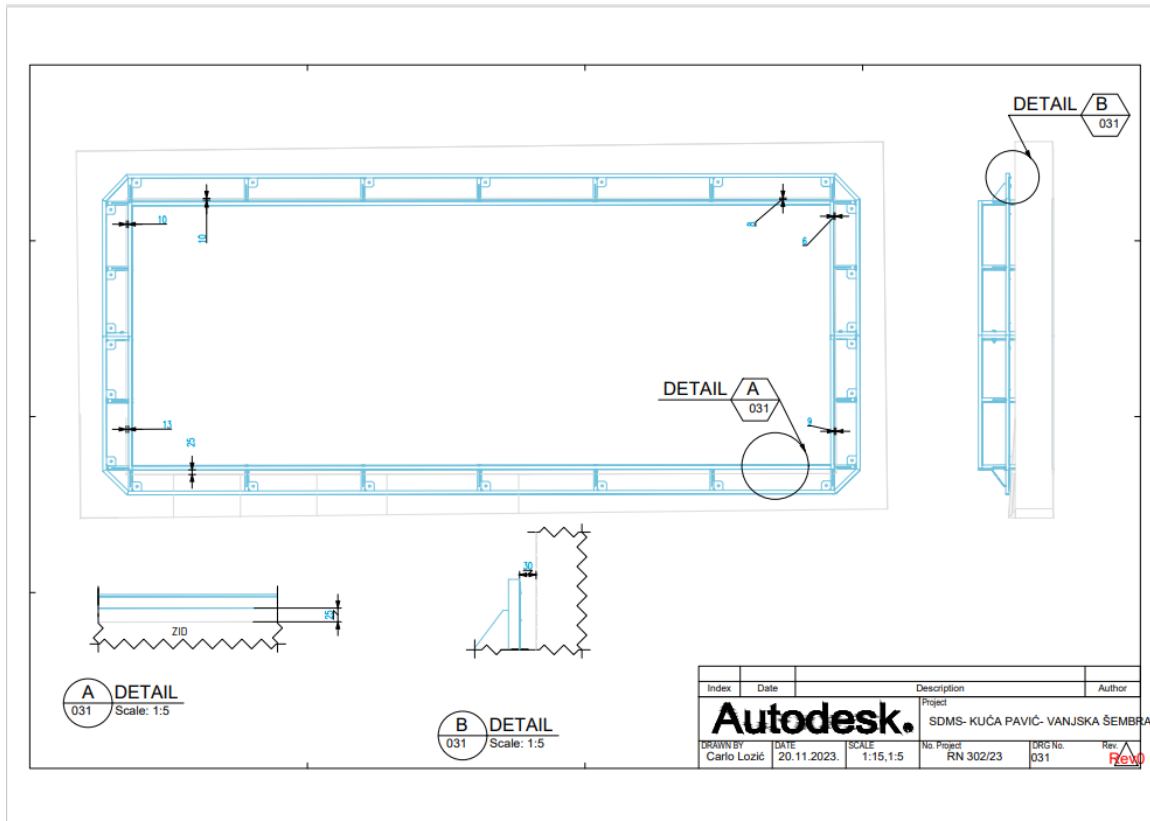
Slika 21. Prikaz montažnog nacrtca
