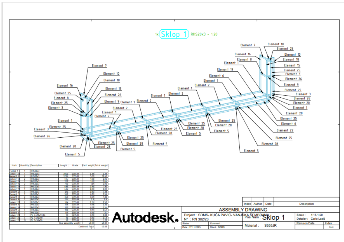
Slika 22. Prikaz sklopnog nacrtca 1/2
