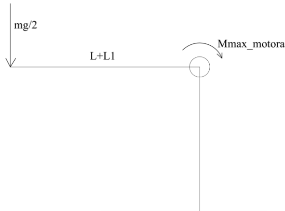
Slika 19. Kritični slučaj za određivanje maksimalne mase
