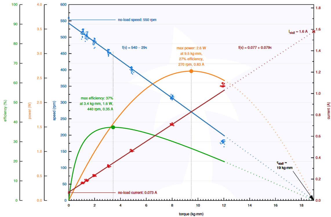
Slika 16 Karakteristika Pololu 12V CB motora
