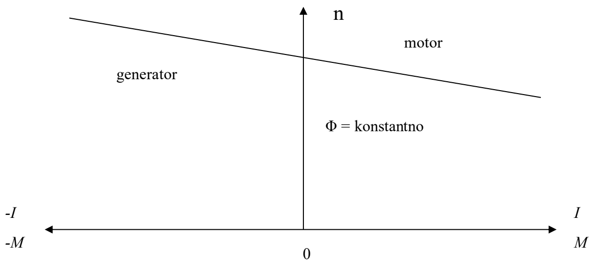
Slika 7 Graf mehaničke karakteristike motora
