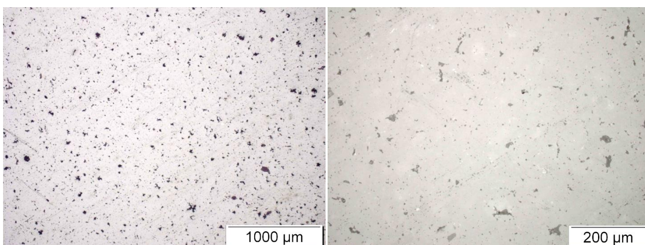
Slika 34. Površina nakon poliranja dijamentnom pastom veličine abraziva 1 µm
