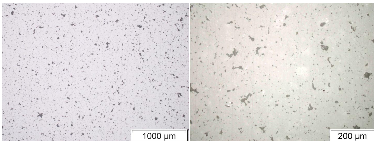
Slika 33. Površina nakon poliranja dijamentnom pastom veličine abraziva 15 µm
