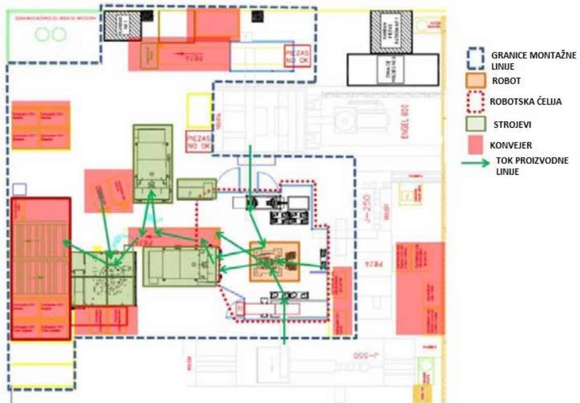
Slika 34. Tlocrt poluautomatske proizvodne linije [68]
