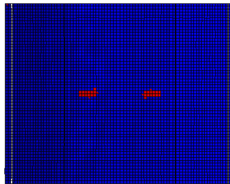
d) Puck-ov kriterij (SDV 10 – popuštanje između vlakana za \sigma_n > 0 )
