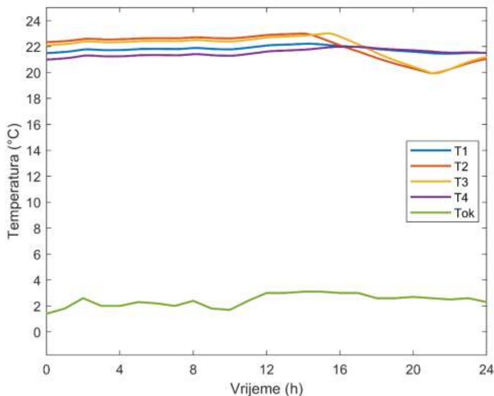
Slika 16. Temperaturni profili zona kućanstva za zimski dan
