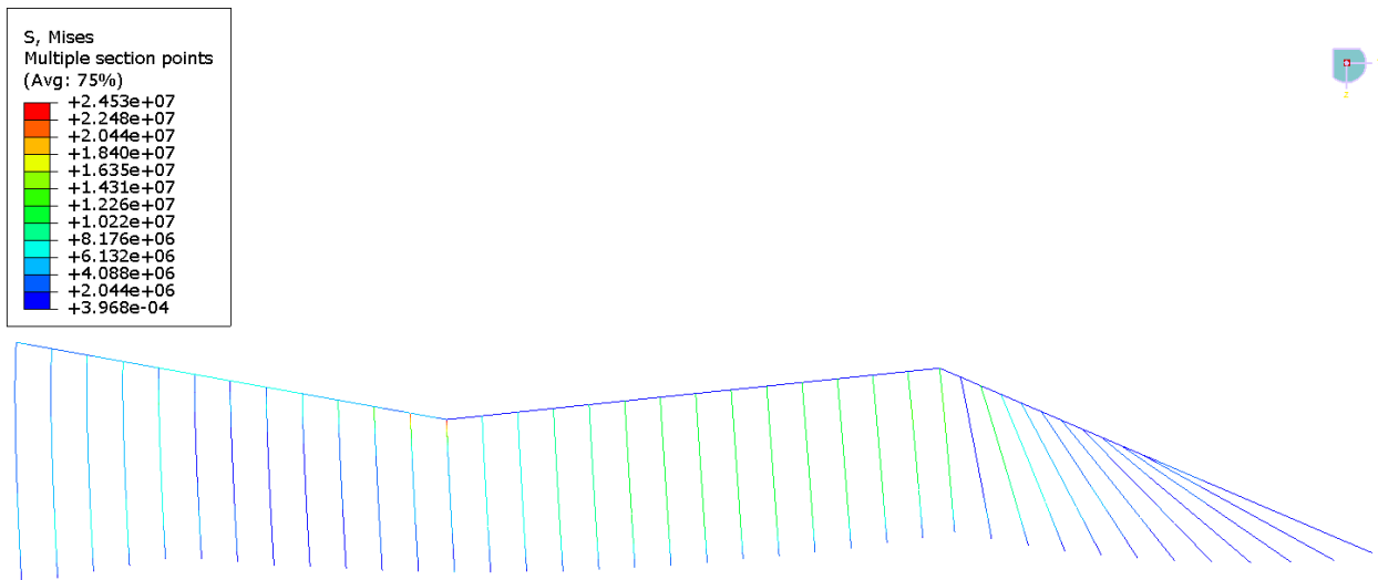
Slika 6.3.4 Napreznja krila u grednim elementima drugog tehničkog sustava [Pa]
