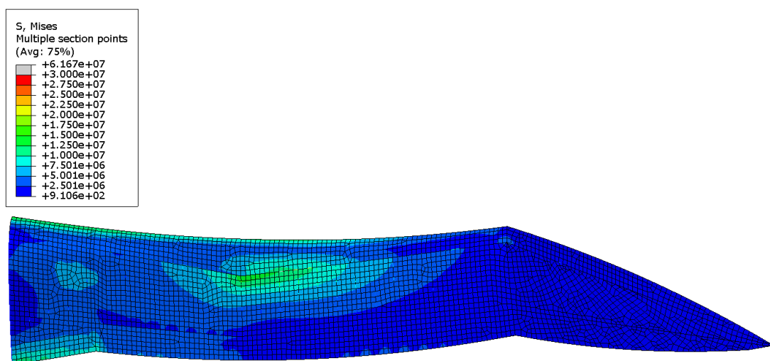
Slika 6.4.1 Ekvivalentno napreznje stvarnog krila prema V.Mises-u [Pa]
