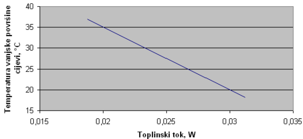
Dijagram 4-Izmjena topline konvekcijom između cijevi i okoline
