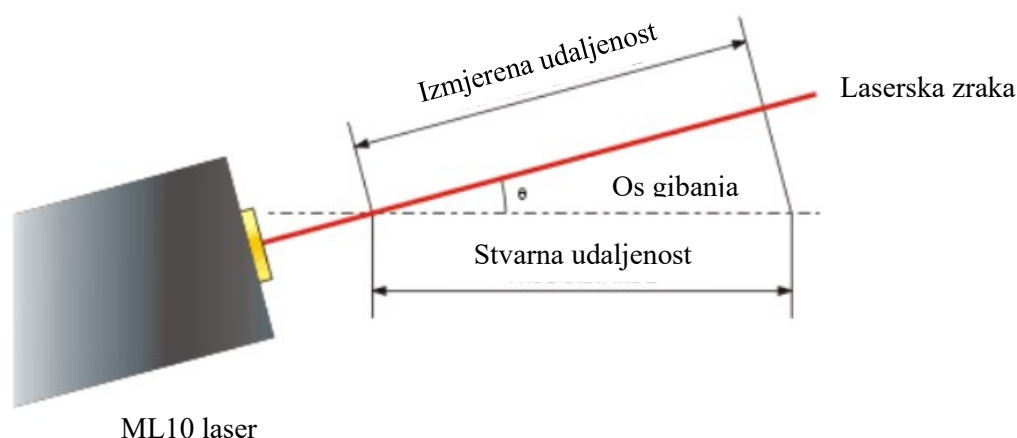
Slika 3.2 Kosinusna pogreška [2]
