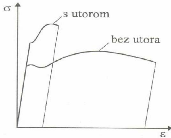
Slika 2.5 Dijagram naprezanje-istezanje
