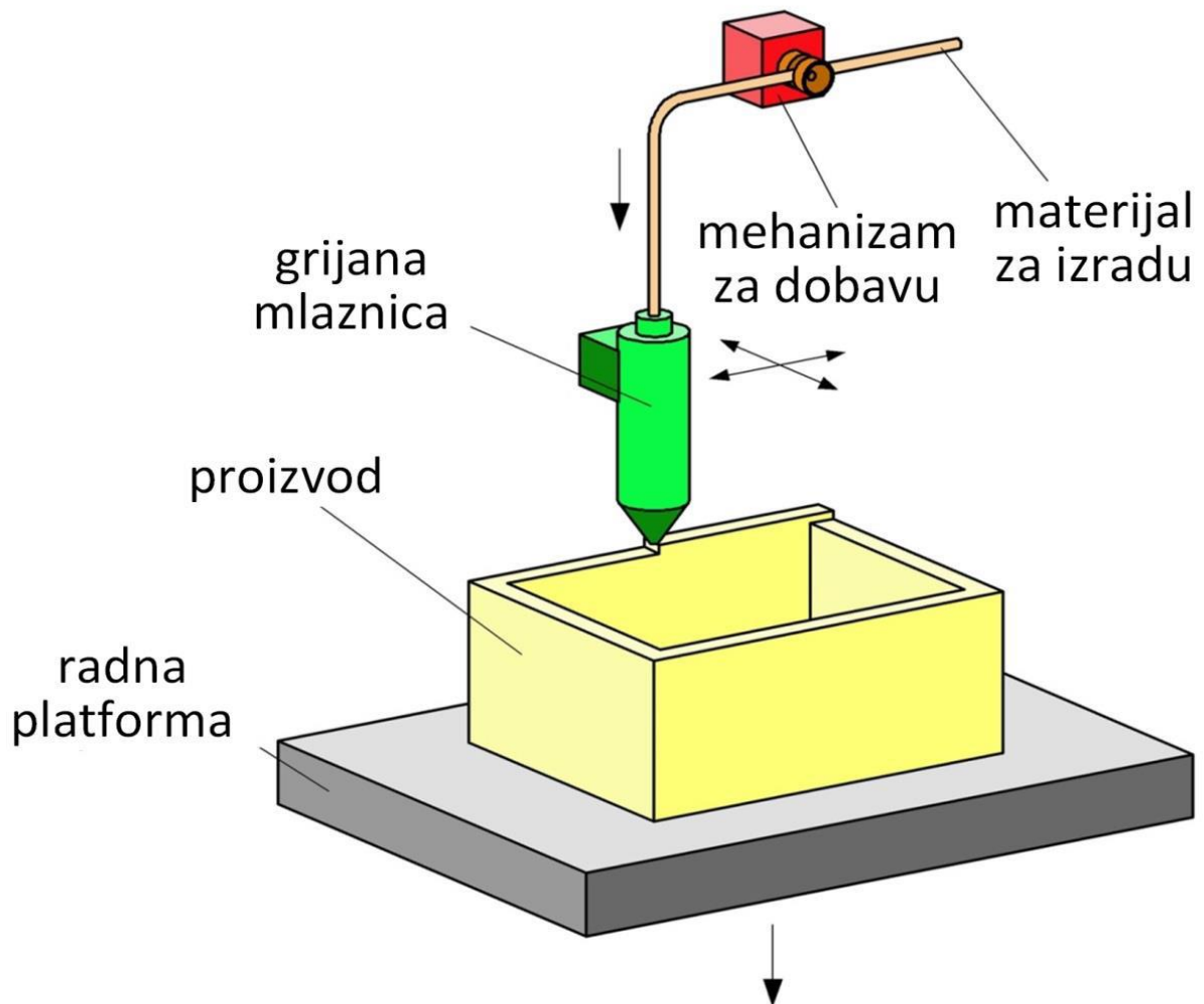
Slika 34. FDM postupak [23]
