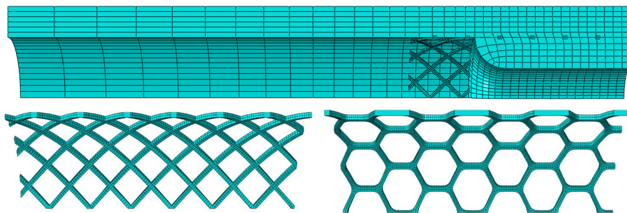
Slika 20. Mreže C3D8H elemenata za stijenkicu s plakom, konvencionalni i Favus-O stent
