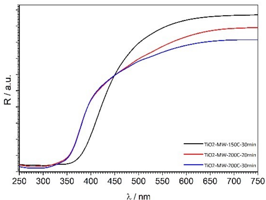
Slika 35. Refleksijski spektar sintetiziranih uzoraka \text{TiO}_2 na temperaturi 150\text{ }^\circ\text{C} tijekom 30 min ( \text{TiO}_2\text{-MW } 150\text{C } 30\text{ min} ) i na temperaturi 200\text{ }^\circ\text{C} tijekom 20 min ( \text{TiO}_2\text{-MW } 200\text{C } 20\text{ min} ) te 30 min ( \text{TiO}_2\text{-MW } 200\text{C } 30\text{ min} )
